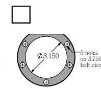
Mopar H1147
